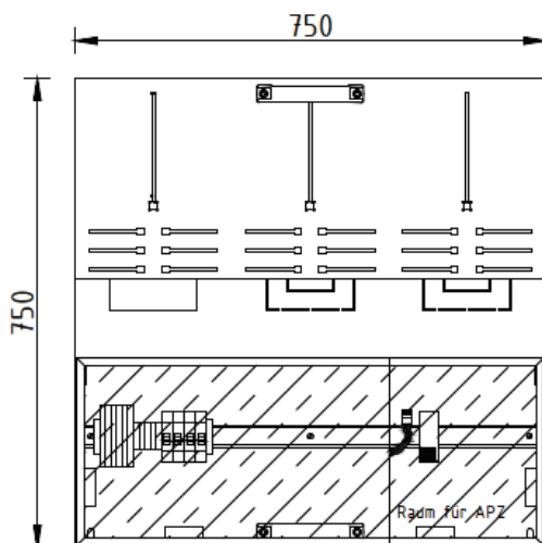
Abbildung Isoliermontageplatte
